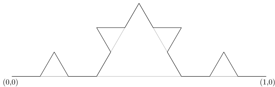
Figure I.7 – Construction de la courbe de Von Koch
