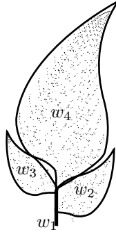
Figure I.13 – Esquisse des transformations qui codent la feuille de fougère
