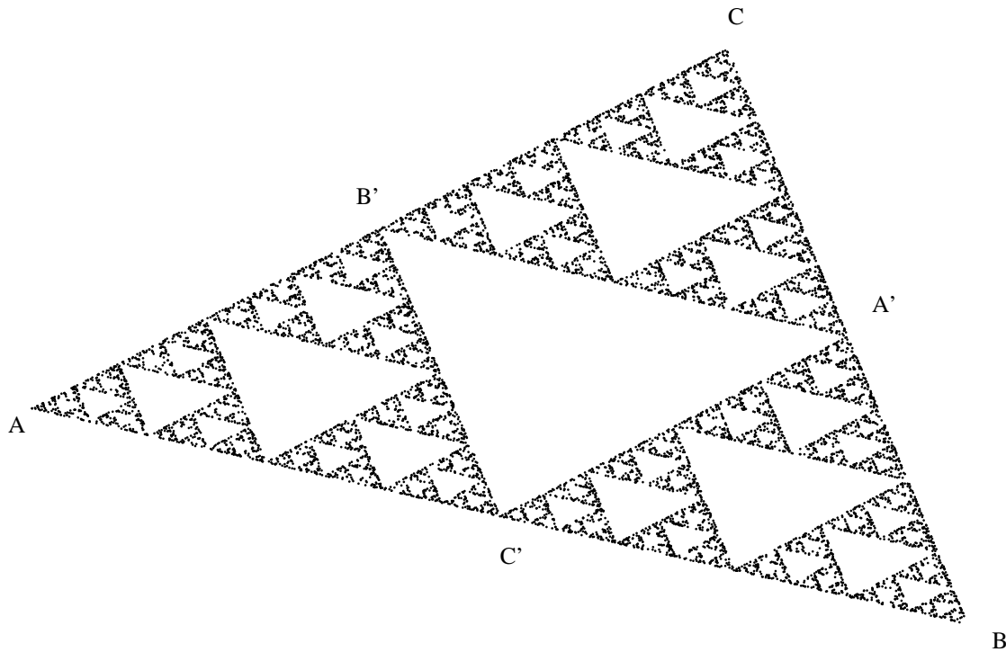
Figure I.6 – Le triangle de Sierpinski, dessiné à l'aide de la méthode des I.F.S.
