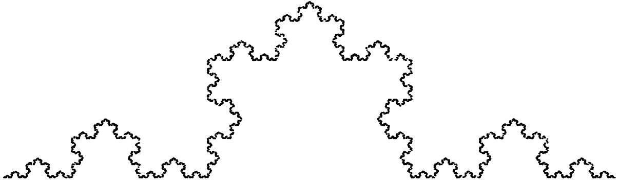
Figure I.8 – La courbe de Von Koch, dessinée à l'aide de la méthode des I.F.S.
