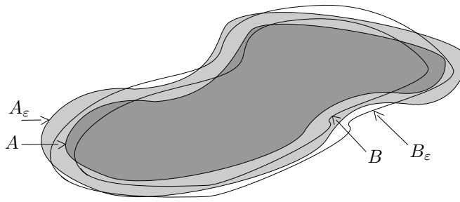
Figure I.10 – La distance de Hausdorff de A à B est inférieure à \varepsilon
