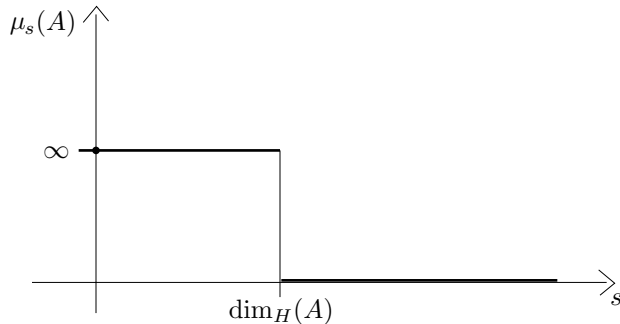
Figure I.9 – Comportement de la s -mesure de A selon les valeurs de s
