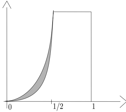
Figure I.3 – L’aire hachurée représente la distance pour la norme \| \cdot \|_1 entre 2 termes de la suite f_n(t)
