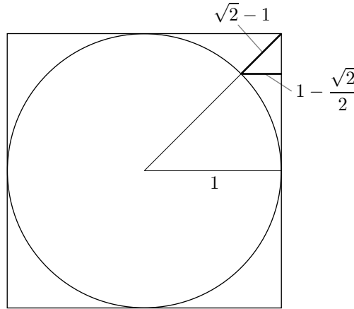
Figure I.11 – Distance de Hausdorff du carré au cercle inscrit
