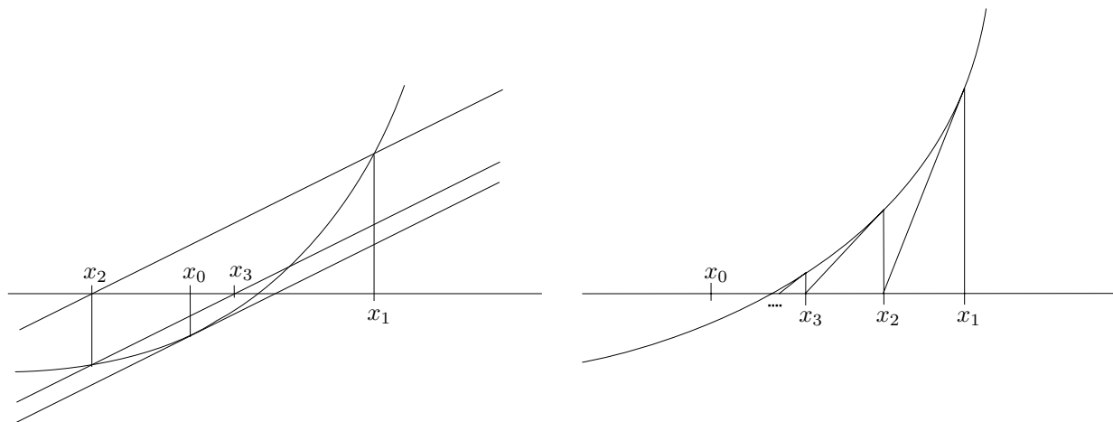
Figure I.4 – Méthode de Newton selon 4.2 et selon 4.3
