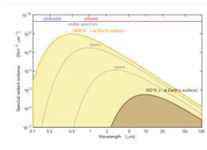
« Spectral radiance of Sun and Earth » von Henriette Sudhaus ist lizenziert unter CC BY-SA
