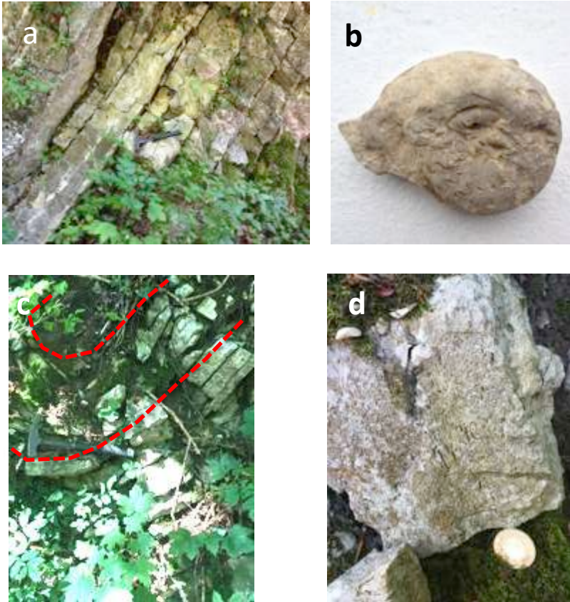
Figure 10: de l'arrêt 3 à l'arrêt 4: a) couches de Plattenkalk inclinées vers le Sud; bordure de la route forestière sur le versant gauche du ruisseau d'Asp («Asper Bach», fig. 7a). b) Ceratite (Ammonite du Trias) du Muschelkalk trouvé dans le Plattenkalk. c) Plis (plis par cassure) dans le Plattenkalk exposé sur le talus de la route forestière. d) Trochitenkalk; les débris de crinoïdes de la forme de petites pièces de monnaie et d'un diamètre de 5 à 10 mm apparaissent soit par altération, soit à la cassure de la roche au marteau.
