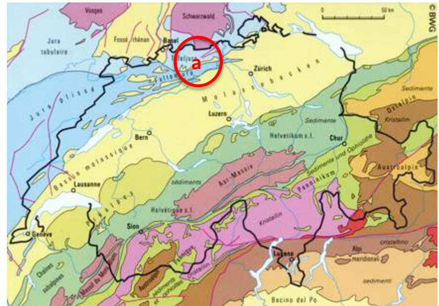
Figure 1 en bas: schéma géologique de la Suisse (source: swisstopo). haut: coupe géologique simplifié du Jura argovien (W. Wildi, simplifié d'après www.Nagra.ch).
