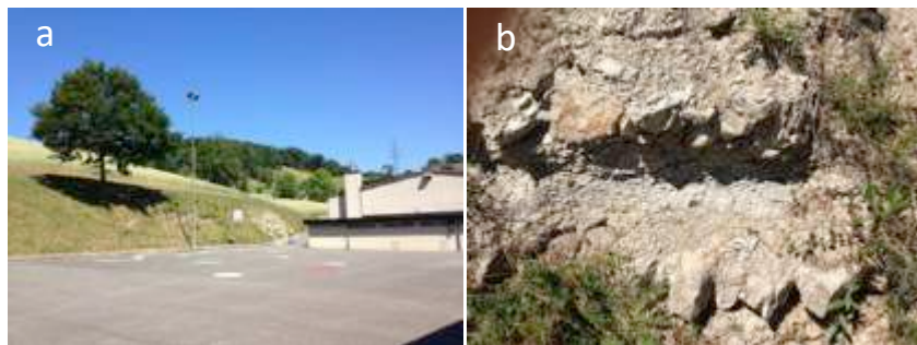
Figure 12: a) Affleurement de Marnes d'Effingen au bord du terrain de sport de l'École de Densbüren. b) Zoom sur une séquence de marnes et marno-calcaires (hauteur du champ: env. 40 cm).
