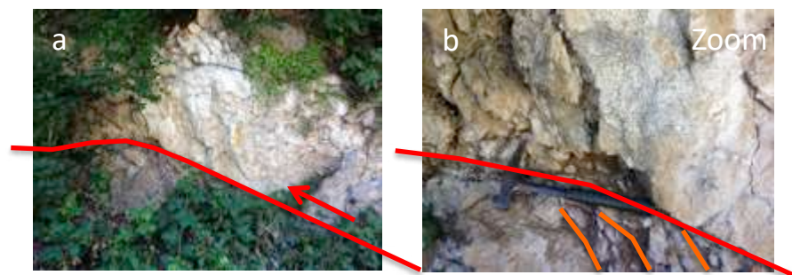
Figure 13 : Chevauchement au sein des calcaires du Dogger le long de la route forestière près du bureau postal de Densbüren (coord. 646 236/256 335)
