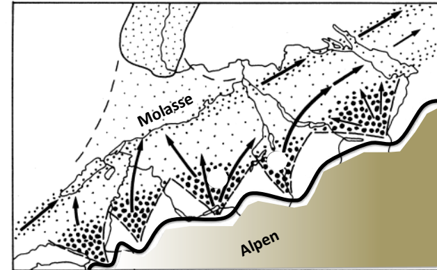
Figure 3: Paléogéographie du front alpin au Fossé rhénan au cours du Paléogène (R. Trümpy 1980). De grands cônes alluviaux amènent le matériel terrigène érodé dans les Alpes vers le bassin molassique.
